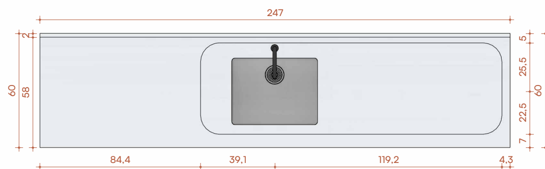
2 Elevação de topo Escala: 1 : 20
